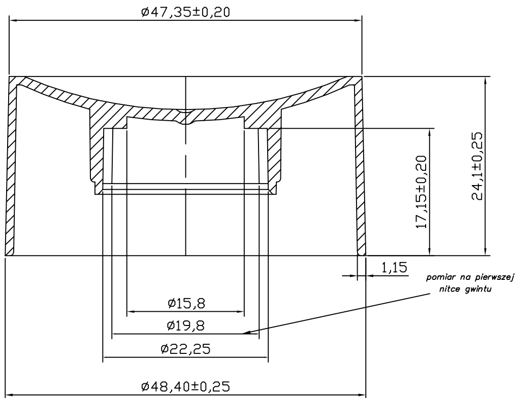
1. GwintTr 22x3
