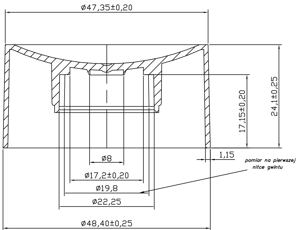
1. GwintTr 22x3
